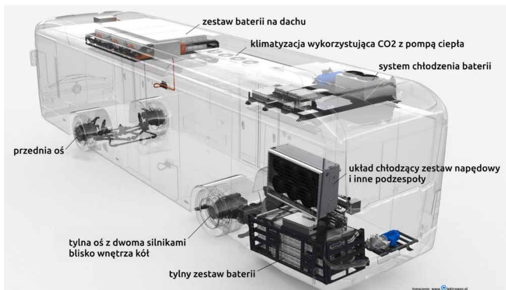
Rysunek 1. Schemat budowy autobusu elektrycznego
